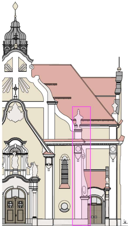
Ansicht West
