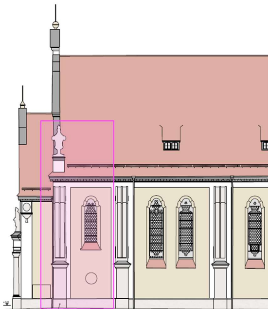
Ansicht Süd
